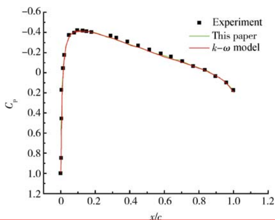
图3 NACA 0012 翼型 0^\circ 攻角下压力系数分布
