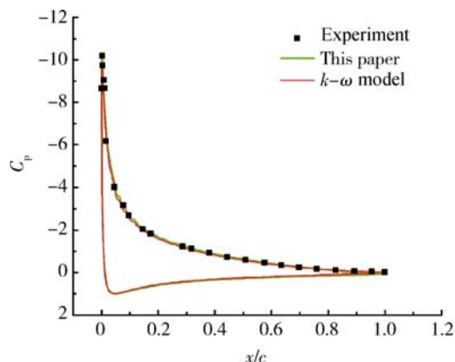
图5 NACA 0012 翼型 15^\circ 攻角下压力系数分布
