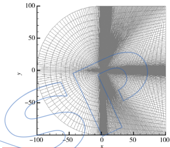
图 8 NACA 4412 流场计算网格
