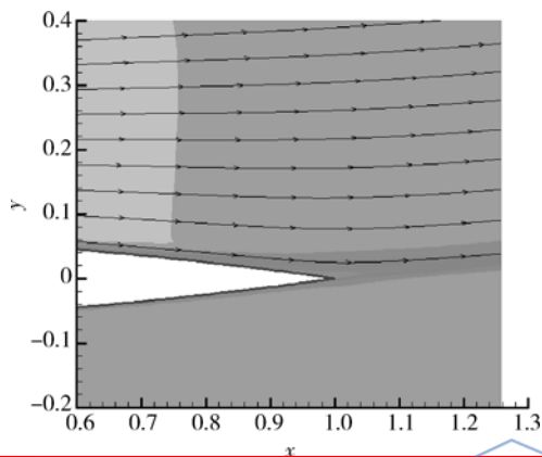
图 6 10^\circ 攻角时翼型尾缘处流线图
